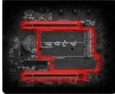
PCIE GEN 5.0 X16 SLOTS & GEN 4.0 M.2 SLOTS
